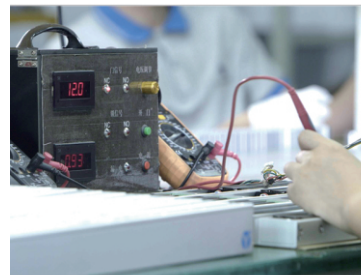
06. 磁力锁功能检测设备 (确保每件产品的各项性能指标100%合格)
