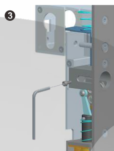
保持調節後鎖舌方向，螺絲鎖緊鎖舌
