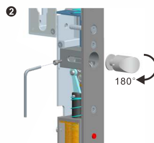
拆下螺絲，鎖舌軸向旋轉180度
