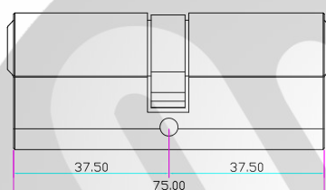
雙開鑰匙雙鎖膽
