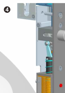
調節後鎖舌方向
